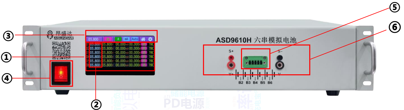
图 2.2.1 ASD 9610H 前面板
